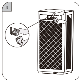
④ 从旧传感器模组上拔出接线端子并换上新的传感器模组。
