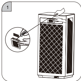
① 用“—”字螺丝刀撬开传感器盖。
